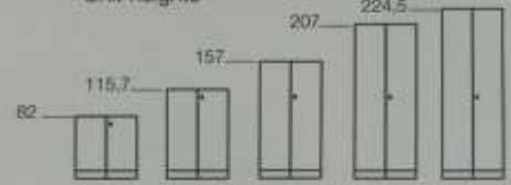
Elementhöhen Unit heights
