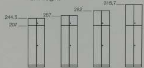
Elementhöhen Unit heights
