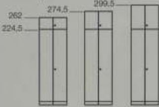
Elementhöhen Unit heights
